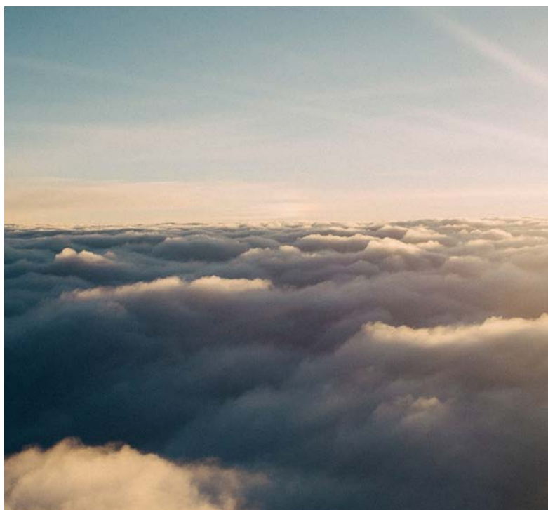
Ozon nás chrání před škodlivým ultrafialovým zářením.
